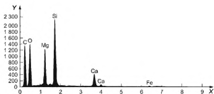
д) Тремолит (без покрытия золотом)
