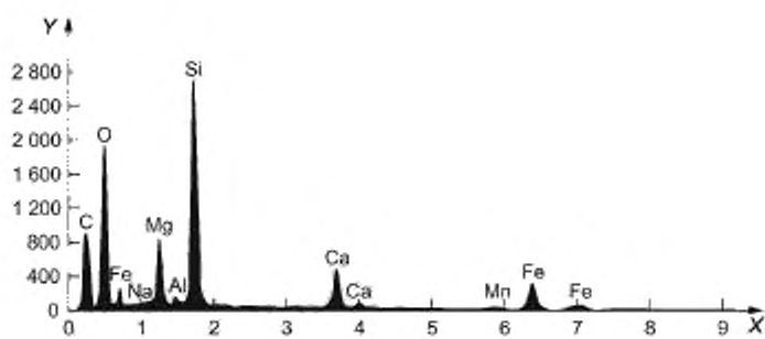
е) Актинолит (без покрытия золотом)
