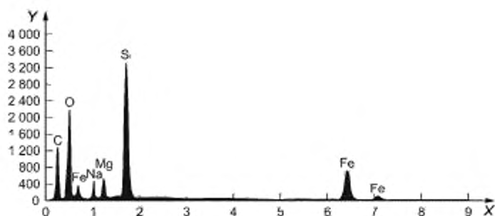
с) Кроцидолит (без покрытия золотом)
