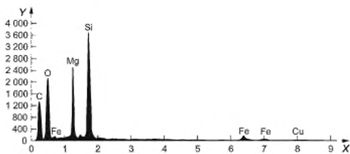
ф) Актофиллит (без покрытия золотом)
