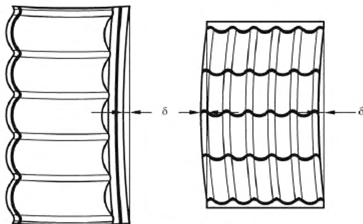
Рисунок 6 — Серповидность
