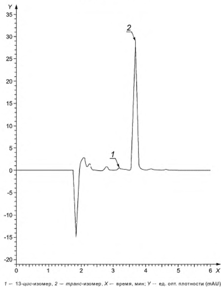
Рисунок А.1 — Хроматограмма градуировочного раствора ретинола пальмитата
