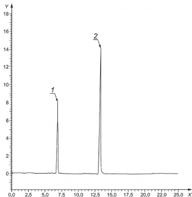
Рисунок А.5 — Хроматограмма градуировочного раствора смеси \alpha -токоферола ацетата и \alpha -токоферола
