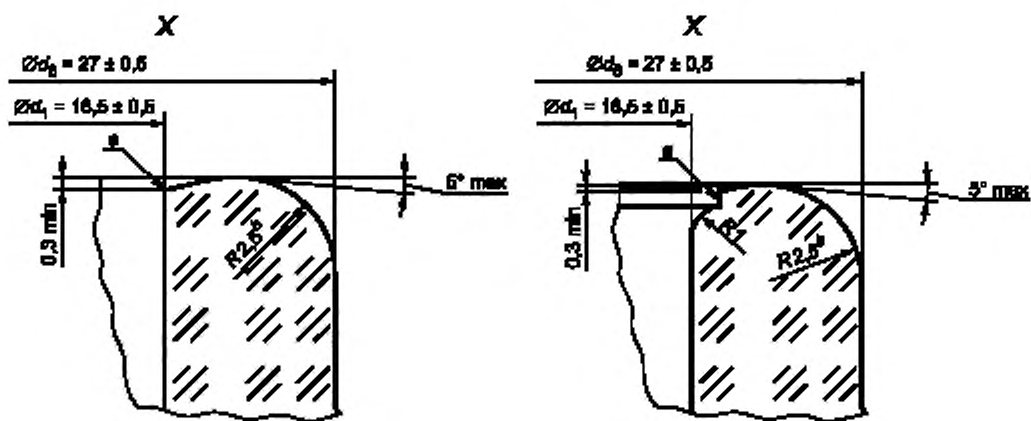
Рисунок 2 — Деталь горловины X
