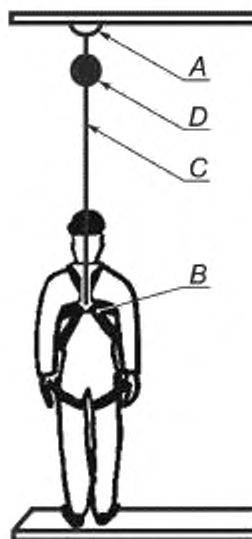
A — анкерная точка, B — страховочная привязь; C — втягивающийся строп (отдельная деталь средства защиты втягивающего типа); D — страховочное устройство (средство защиты втягивающего типа)
