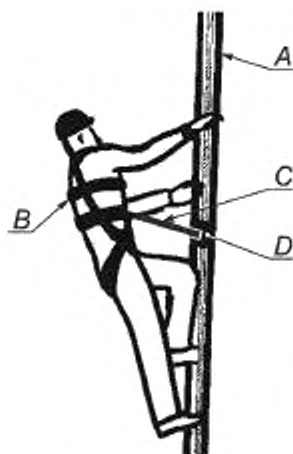
A — жесткая анкерная линия; B — страховочная привязь; C — строп, D — устройство ползункового типа
