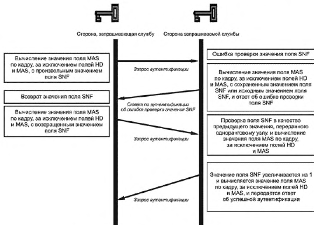
Рисунок 10 — Последовательность инициализации поля SNF
