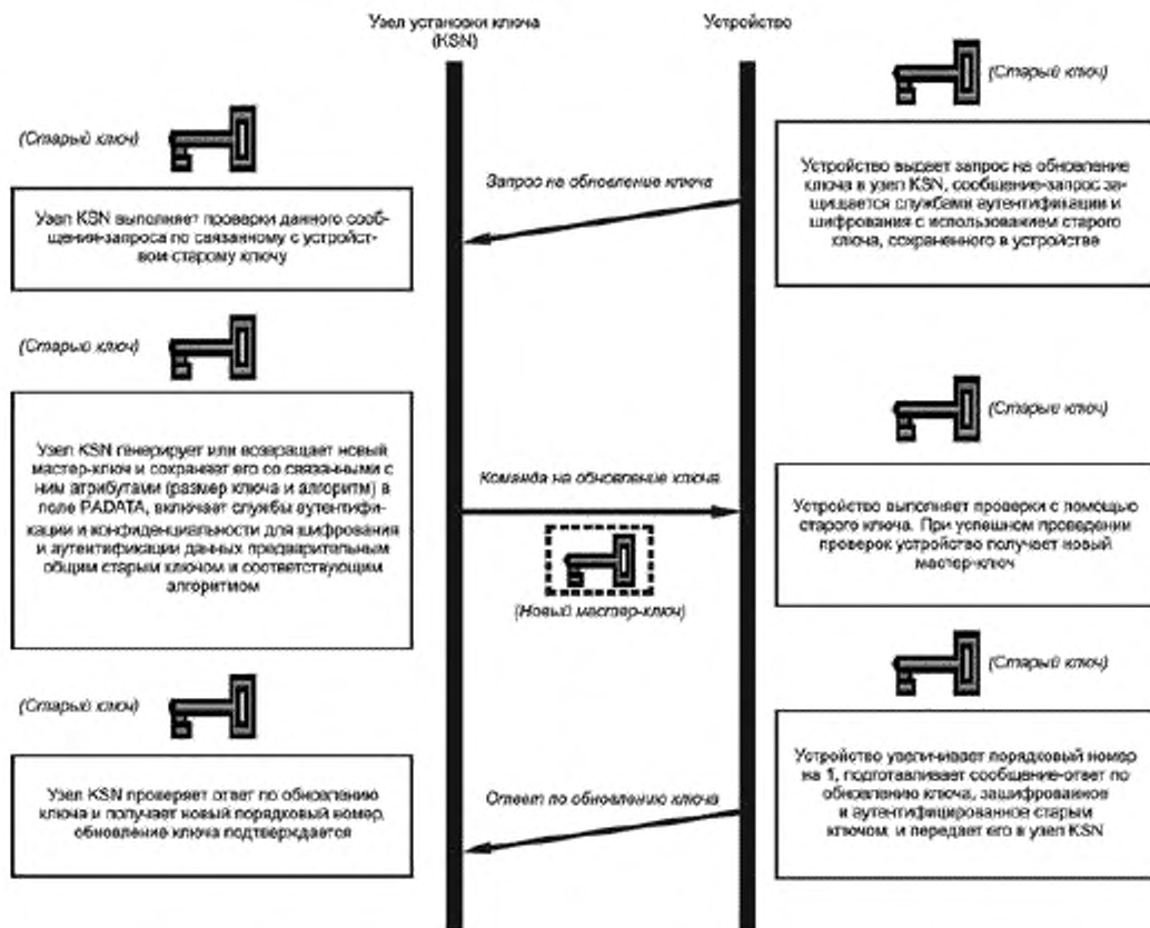
Рисунок 24 — Последовательность обновления мастер-ключа, запрашиваемого устройством
