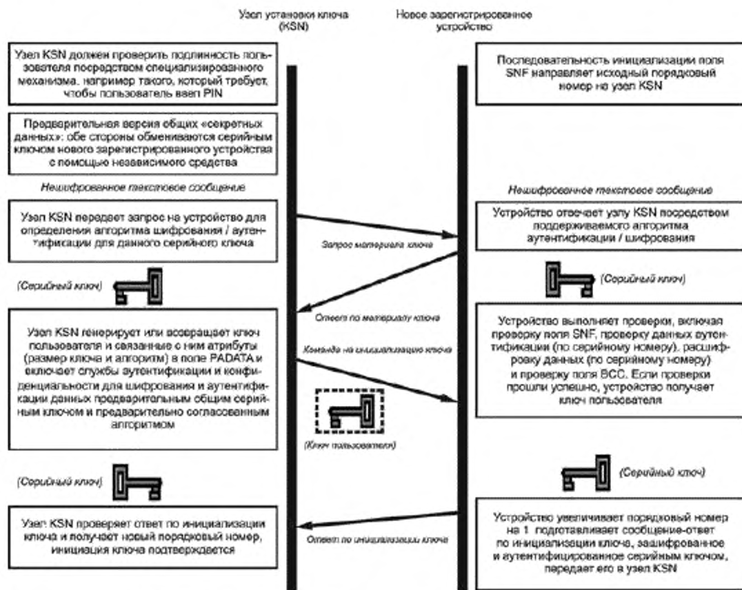
Рисунок 15 — Последовательности инициализации ключа пользователя
