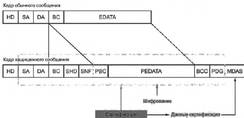
Рисунок 2 — Сравнение кадров обычного и защищенного сообщений
