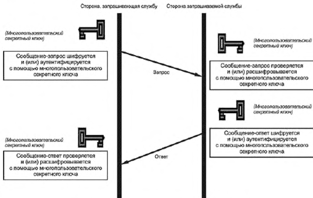
Рисунок 3 — Взаимодействие сторон на основе протокола SCPM
