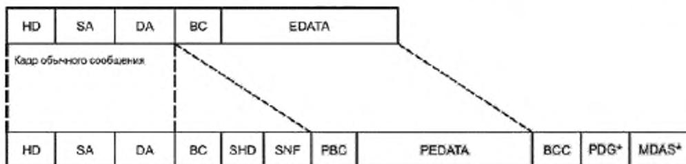
Кадр защищенного сообщения
