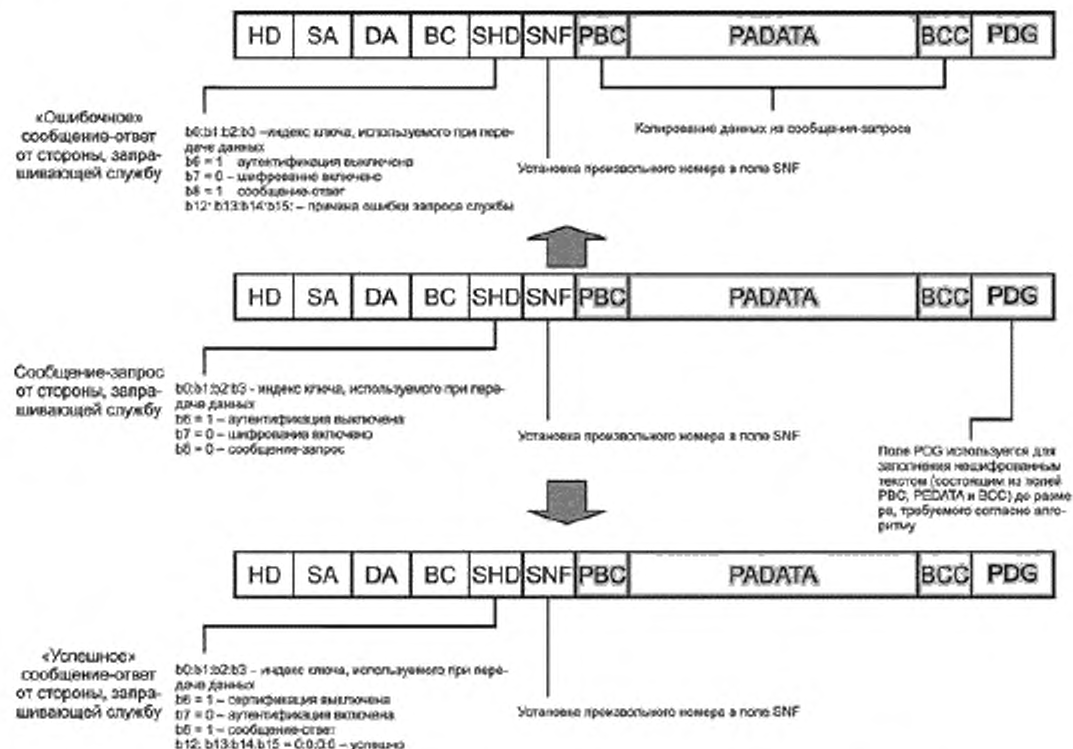
Рисунок 13 — Кадры защищенного сообщения, использующие службу шифрования
