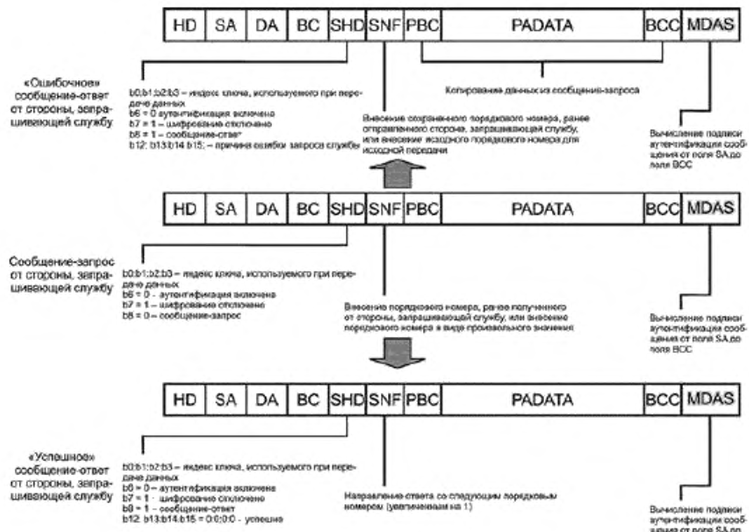
Рисунок 12 — Кадры защищенного сообщения, использующие службу удостоверяющей подписи
