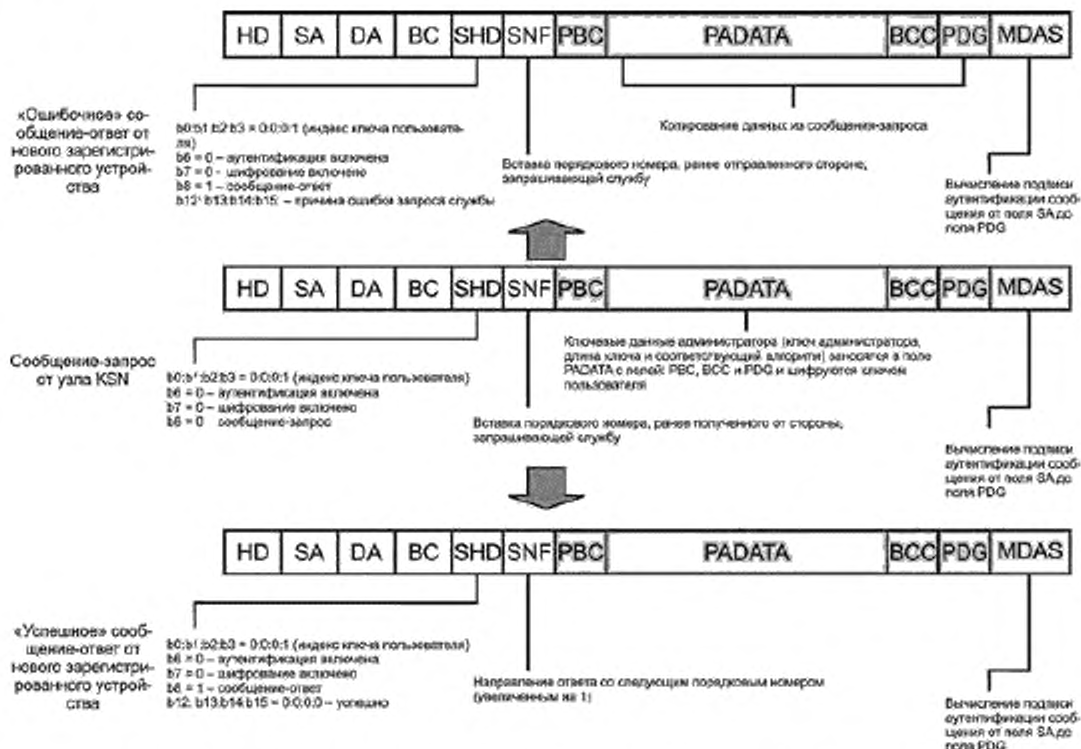
Рисунок 18 — Кадры защищенного сообщения инициализации ключа провайдера услуг
