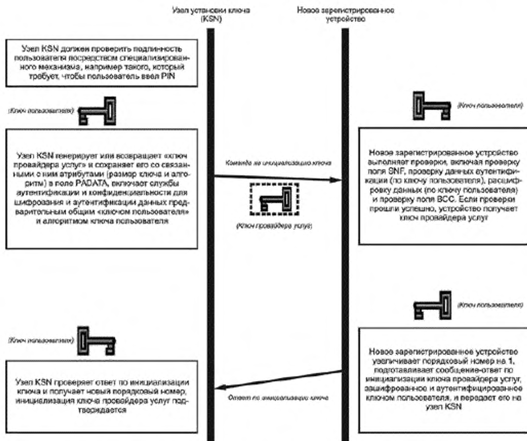
Рисунок 17 — Последовательности инициализации ключа провайдера услуг
