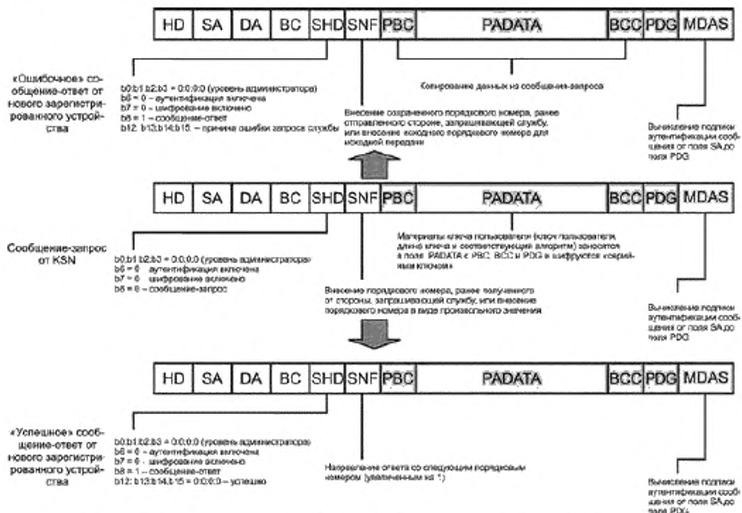
Рисунок 16 — Кадры защищенного сообщения об инициализации ключа пользователя
