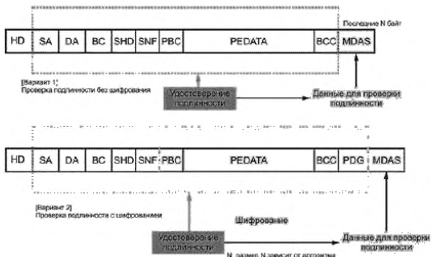
Рисунок 9 — Вычисление данных аутентификации
