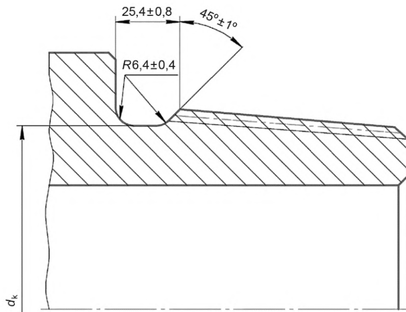
Рисунок 6 — Разгрузочная канавка на nipple-конце
