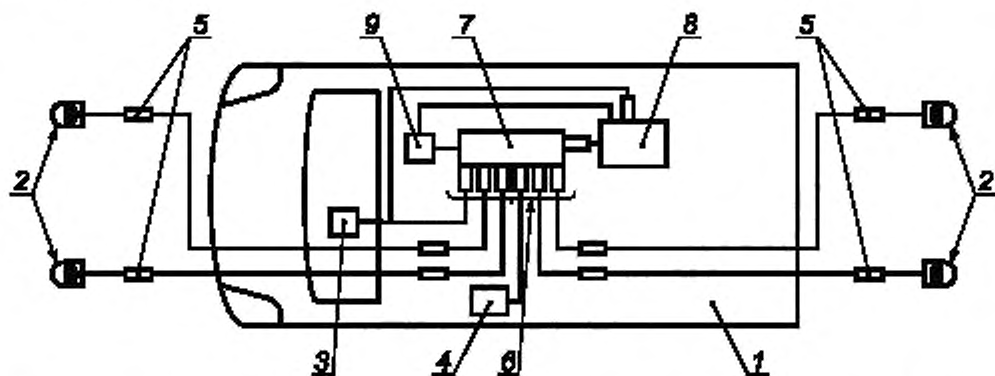
1 — транспортное средство; 2 — фотоприемные устройства; 3 — GPS-приемник; 4 — датчик определения скорости; 5 — герметичные разъемы; 6 — разъемы для подключения к USB-хабу; 7 — USB-хаб; 8 — блок управления; 9 — преобразователь напряжения 12/230 В
