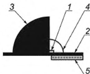
1 — приемная поверхность фотоголовки; 2 — основание; 3 — экран; 4 — защитный колпак; 5 — светодиодная лента, обозначающая габаритные размеры мобильной установки (устанавливают при необходимости)
