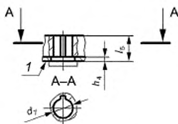
Рисунок 11 — Передача крутящего момента через шпонку
