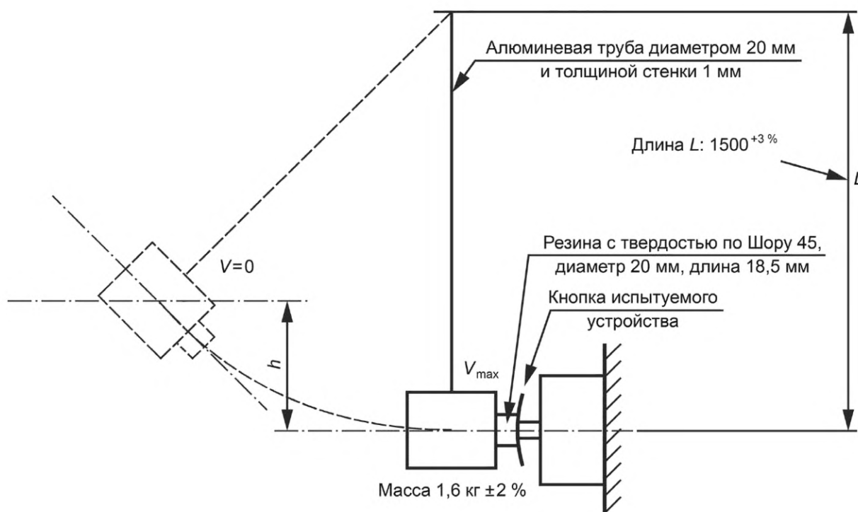
Рисунок 1 — Испытательный боек
