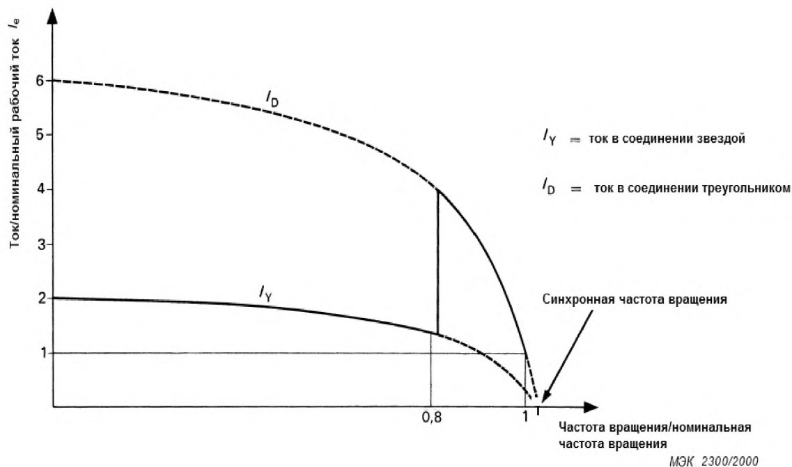
Рисунок 1 – Типичные кривые тока и вращающего момента при пуске по схеме звезда-треугольник (см. 1.1.2.2.1)
