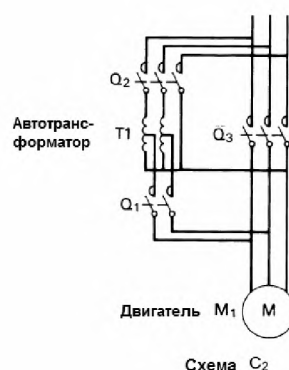
Рисунок 5 – Типичные способы и схемы пуска асинхронных двигателей переменного тока при помощи автотрансформаторов, лист 1
