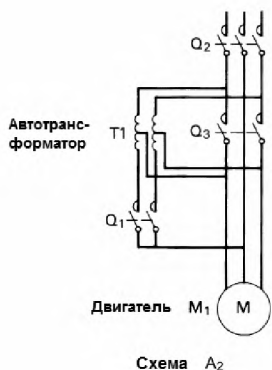
Рисунок 5 – Типичные способы и схемы пуска асинхронных двигателей переменного тока при помощи автотрансформаторов, лист 1
