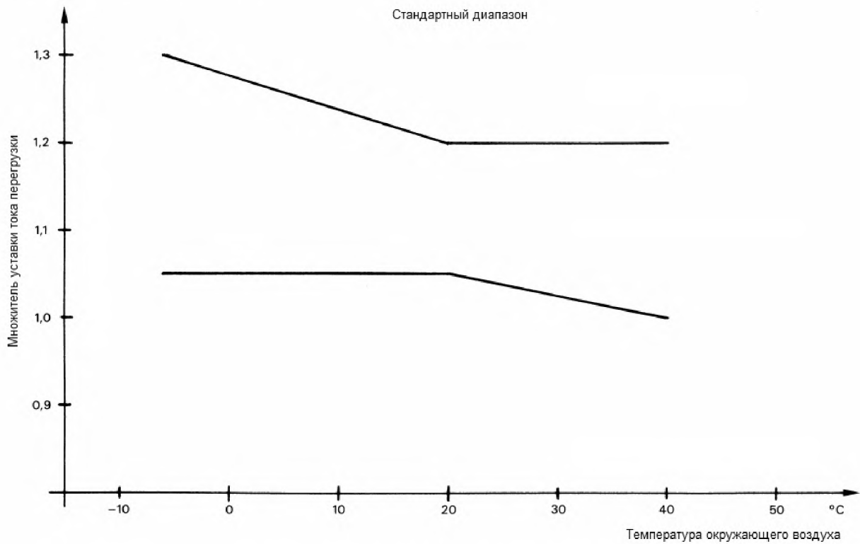
Рисунок 7 – Зависимости пределов кратности уставок тока от температуры окружающей воздуха для компенсированных реле перегрузки с выдержкой времени (см. 8.2.1.5.1)
