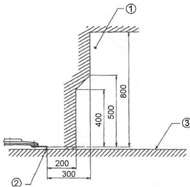
1 – зона расположения защитной скобы; 2 – траектория движения рабочего органа; 3 – почва
