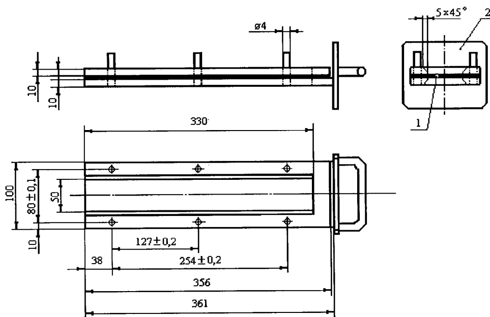
1 – образец; 2 – заслонка
