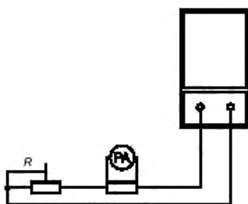
R — балластный реостат; РА — амперметр с шунтом
