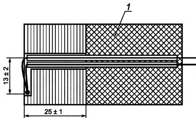
1 — стена испытательного угла
