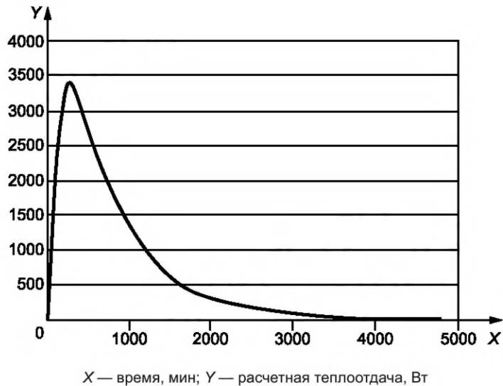
Рисунок С.2 — Расчетная теплоотдача
