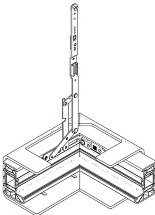
Рисунок Д.3 — Схема испытания по определению прочности крепления ножничной опоры (скрытой верхней петли) на уголке рамы
