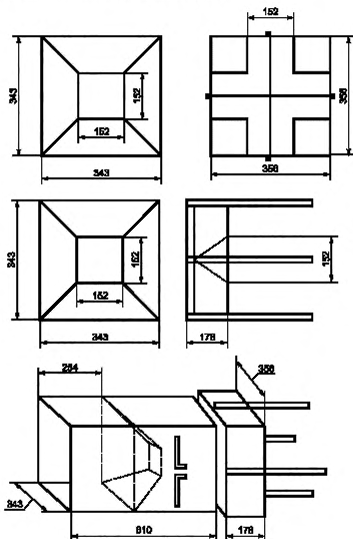
Рисунок А.1 — Схема делителя башенного типа
