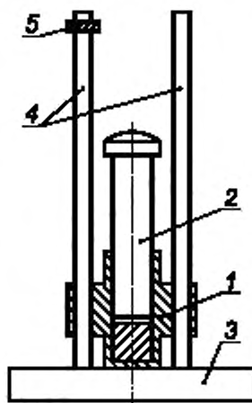
1 — падающий блок; 2 — поршень; 3 — опорная плита; 4 — направляющие стержни; 5 — ограничитель
