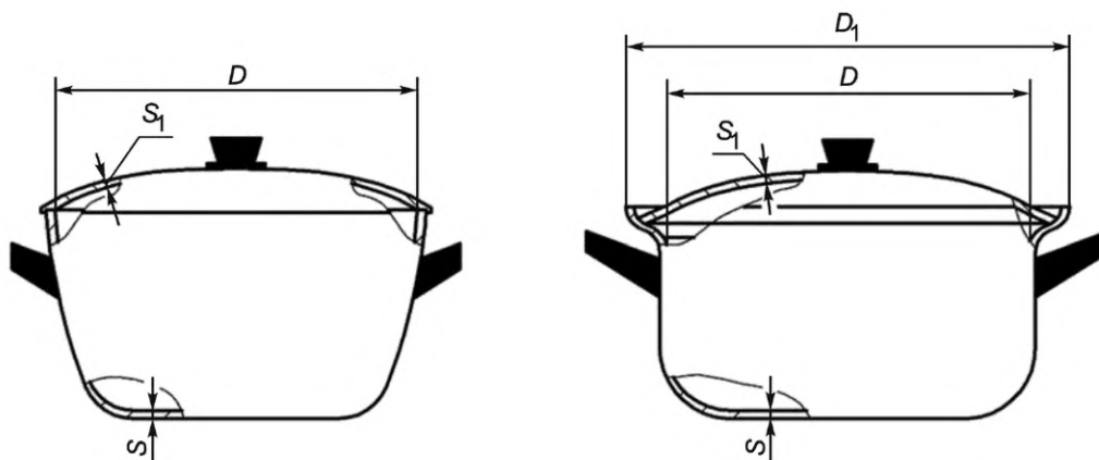
Рисунок 3 — Кастрюля полусферическая
