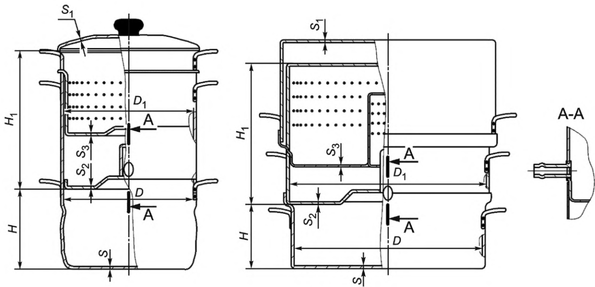
Рисунок 24 — Соковарка
