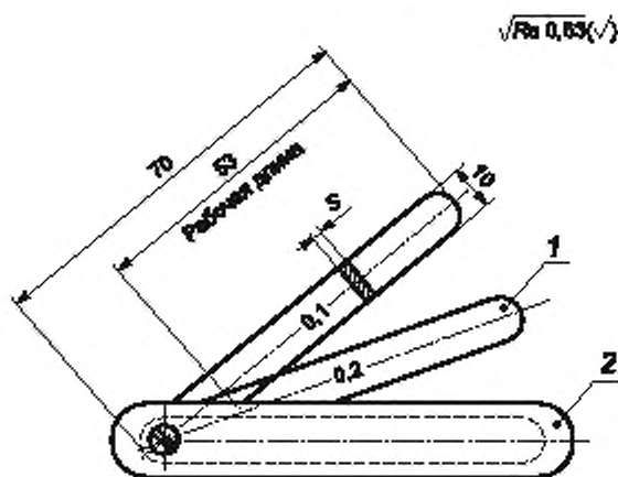
Рисунок А.1 — Набор плоских щупов
