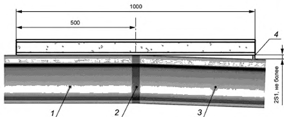
а — Измерение вылуклости стыка по поверхности катания головки рельса (вид сбоку)
