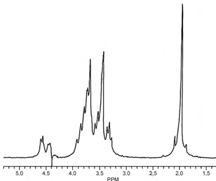
Рисунок 2 — ^1\text{H} ЯМР-спектр гиалуроната из петушиного гребня ( M_w \sim 700\,000 )
