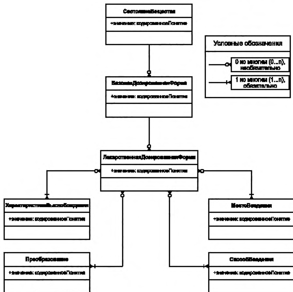
Рисунок 3 — Схема лекарственной дозированной формы с указанием ассоциаций в вилчкообразной нотации
