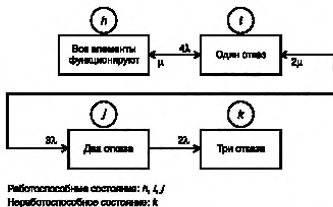
Рисунок В.11 — Диаграмма состояний с группировкой элементов для вычисления показателей безотказности системы, представленной на рисунке В.10
