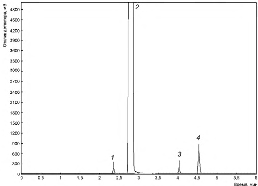
Рисунок 3 — Хроматограмма пробы товарного диэтиленгликоля на капиллярной колонке VERTICAL VertiBond-1
