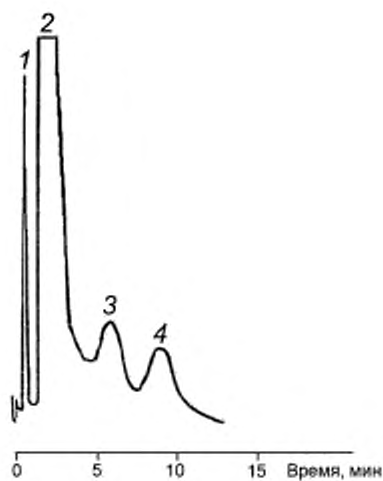
Рисунок 1 — Типовая хроматограмма органических примесей в диэтиленгликоле на колонке с насадкой I
