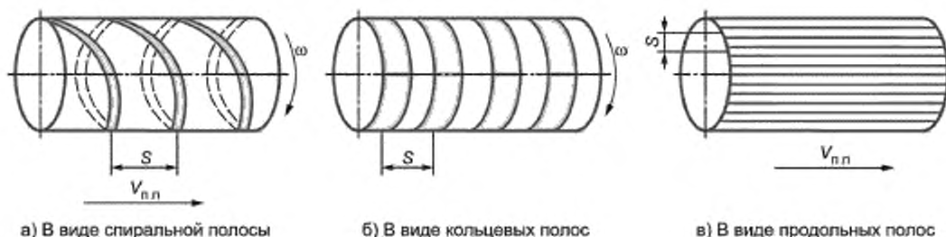
Рисунок 3 — Триботехнические рисунки лазерного термоупрочнения цилиндрической поверхности
