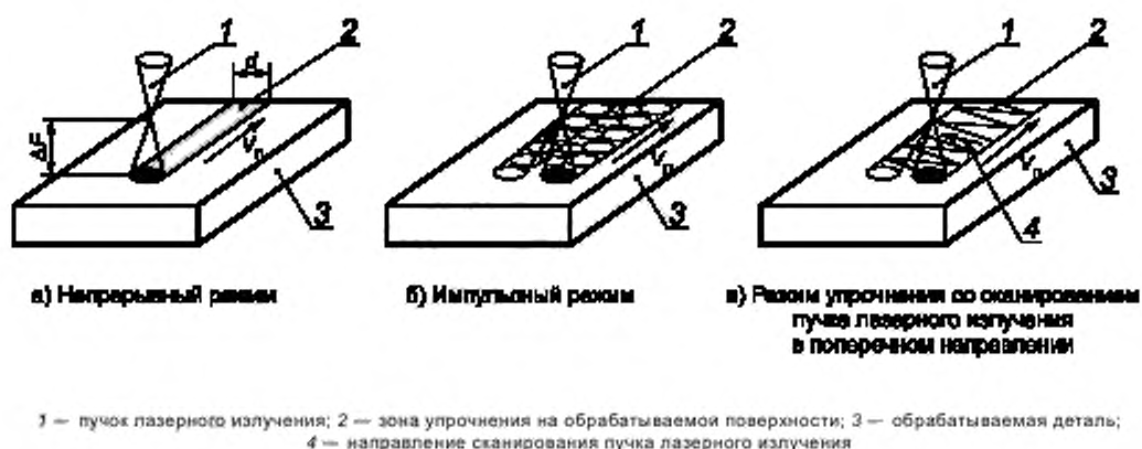
Рисунок 6 — Схемы проведения процесса при различных режимах работы лазера
