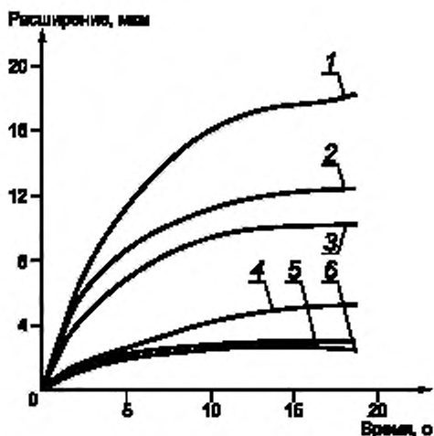
1 — сталь/Au; 2 — Mg; 3 — Al; 4 — Si/Au; 5 — Ag; 6 — Cu
