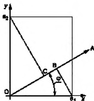
x, y — оси координат абсолютной системы координат; A — направление анализатора; B — точка пересечения перпендикуляра к OA от a_2 с OA , C — точка пересечения перпендикуляра к OA от a_1 с OA ; O — начало системы координат
