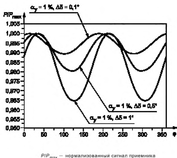
Рисунок А.7 — Влияние разности коэффициентов поглощения и сдвига фазы на сигнал приемника
