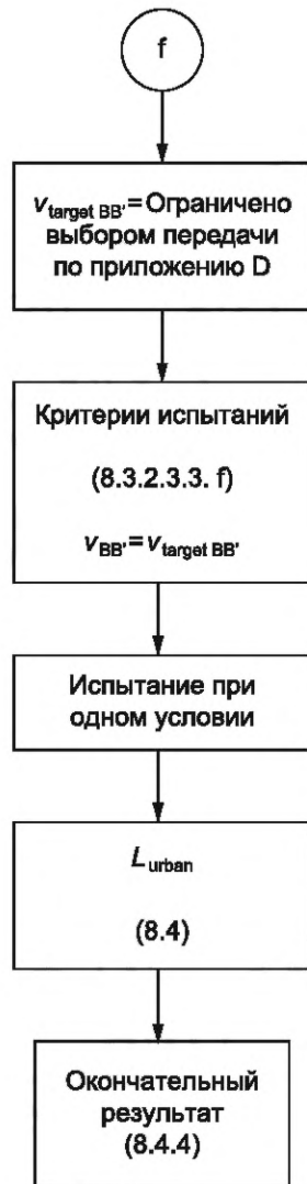
Рисунок Е.2 — Блок-схема для испытаний тяжелых коммерческих автомобилей без фиксирования передач
