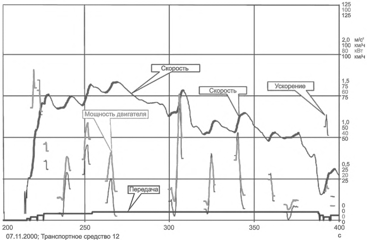
Рисунок А.2 — Пример записи параметров движения одного транспортного средства в зависимости от времени
