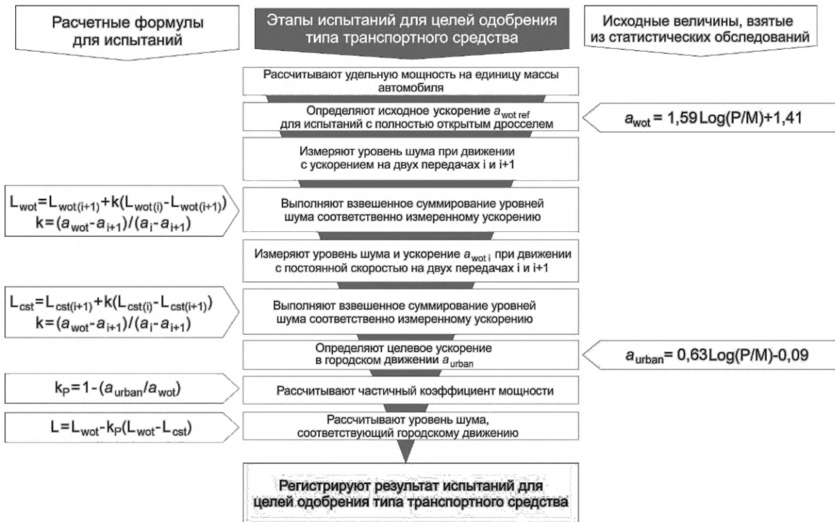
Рисунок А.19 — Методика измерения шума при движении
