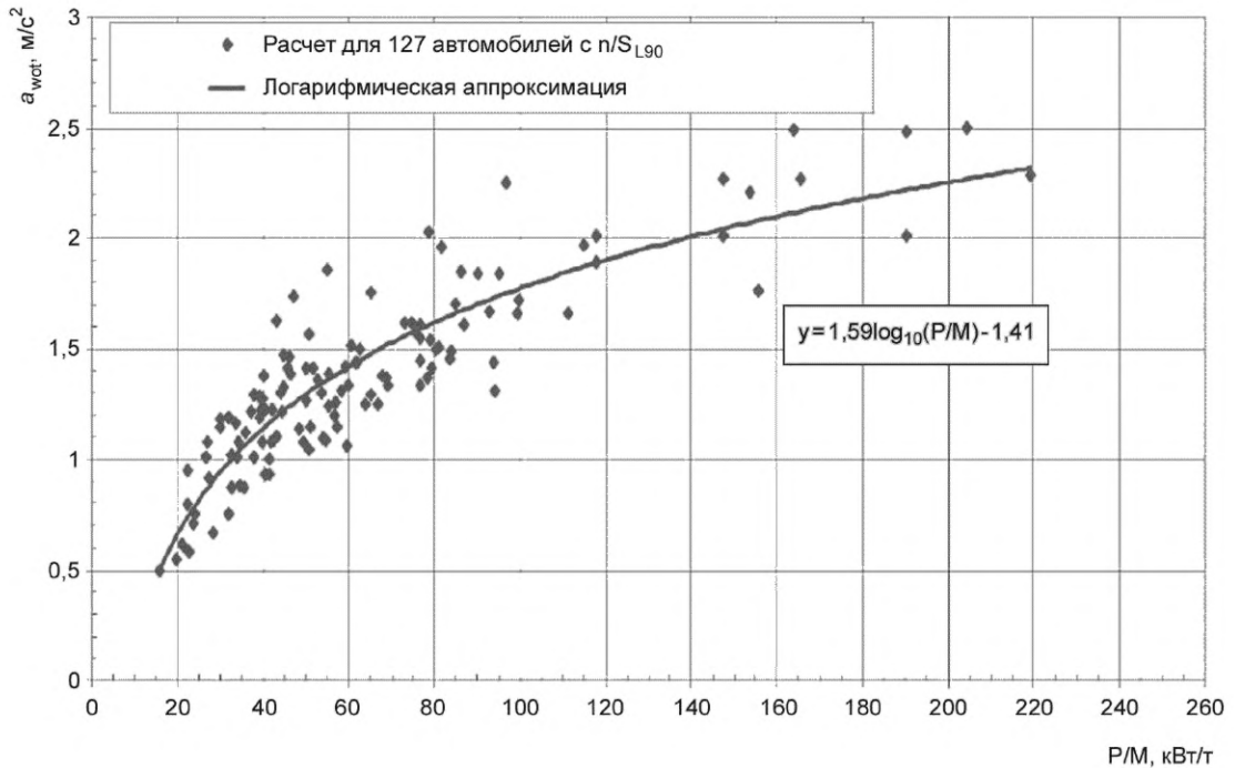
Рисунок А.17 — Регрессионная зависимость a_{wot\ ref} от удельной мощности на единицу массы (для 127 транспортных средств)
