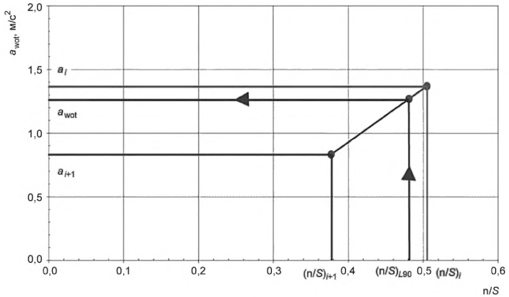
Рисунок А.16 — Определение ускорения a_{wot\ 50} при полностью открытом дросселе
