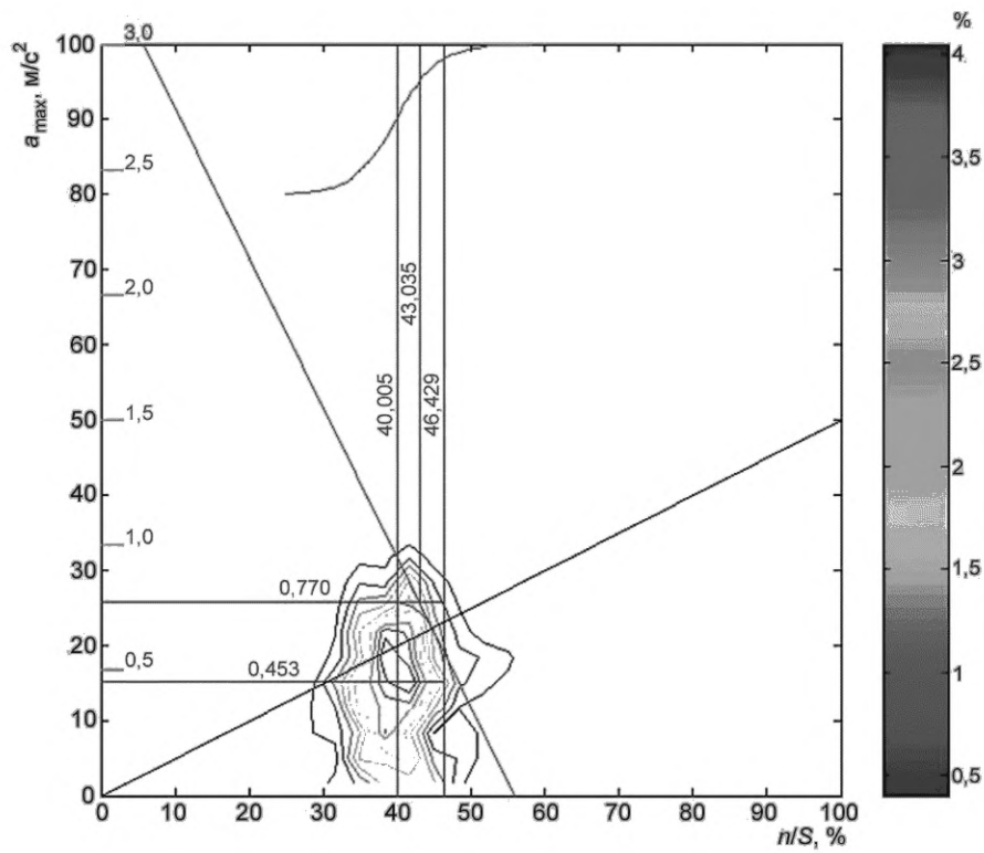
Рисунок А.13 — Определение (n/S)_{L90,a90} при скорости 50 км/ч
