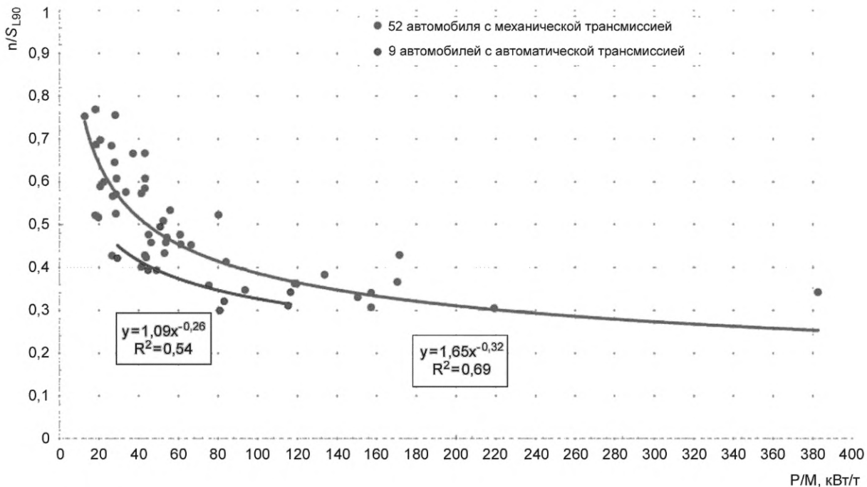
Рисунок А.15 — Скорость двигателя при максимальном ускорении и скорости 50 км/ч — регрессионная кривая [(n/S)_{L90,a90}] при 90-м процентиле уровня звукового давления, 90-м процентиле ускорения и скорости 50 км/ч], как функция удельной мощности на единицу массы (PMR) для 52 транспортных средств
