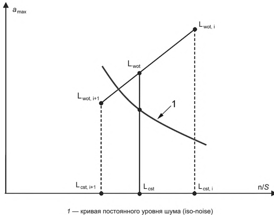
Рисунок А.12 — Кривая постоянного уровня шума
