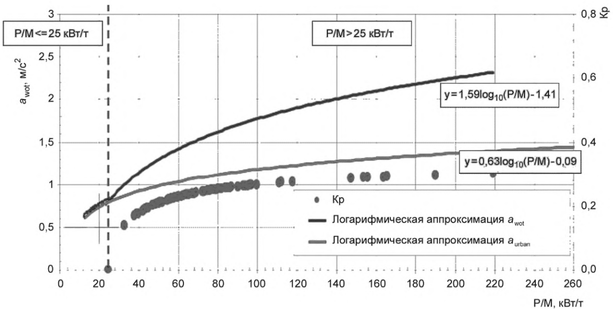
Рисунок А.18 — Коэффициент k_p
