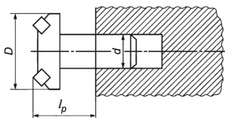
Рисунок 4 — Пример для сборной фрезы
