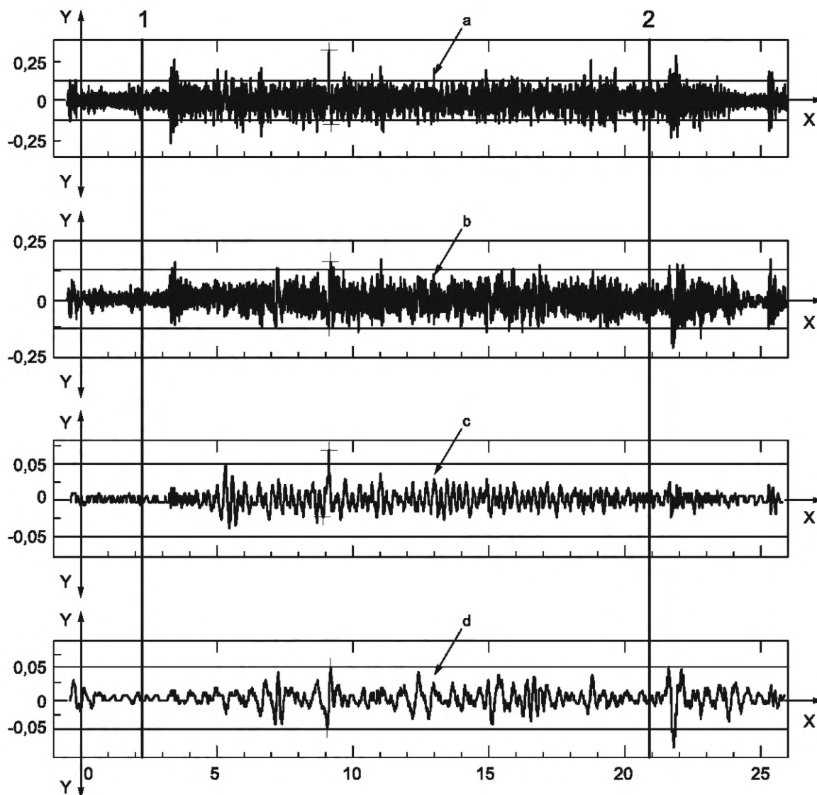
Y — вибрация, m/s^2 ; X — время, с; a — составляющая вибросигнала по координатной оси x (без корректировки); b — составляющая вибросигнала по координатной оси y (без корректировки); c — составляющая вибросигнала по координатной оси x (после корректировки); d — составляющая вибросигнала по координатной оси y (после корректировки)
