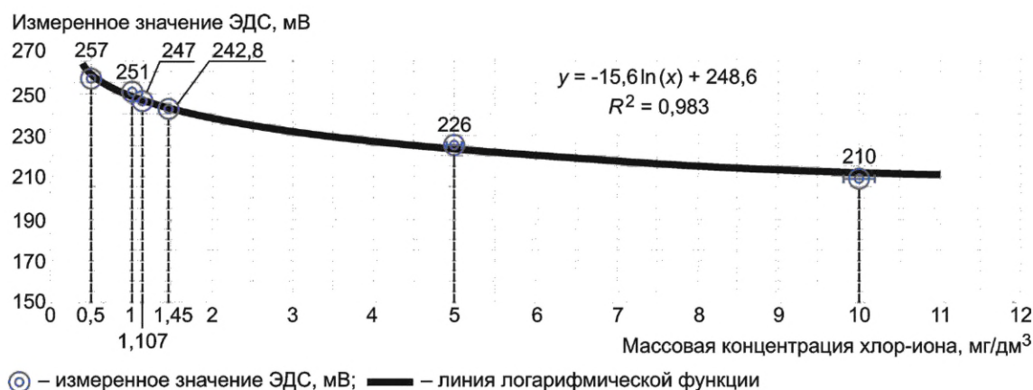
Рисунок В.1 — Зависимость ЭДС (мВ) от концентрации хлор-иона (мг/дм 3 )
