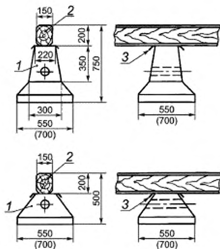
Рисунок А.5 — Опоры фундамента
