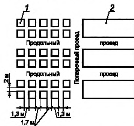
1 — штабель, 2 — группа штабелей
