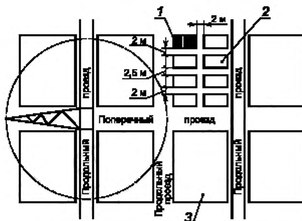
б) Укладка прямо башенным краном
