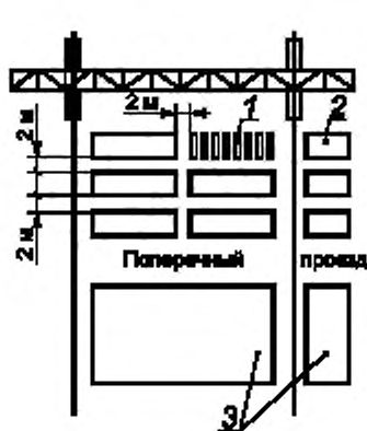
а) Укладка козловым краном
