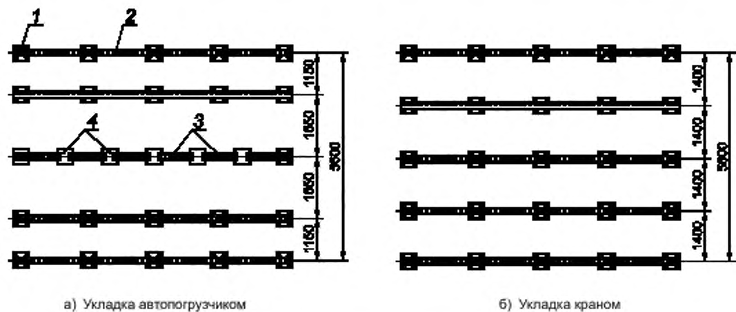
Рисунок А.4 — Схема подштабельных фундаментов для укладки пакетных штабелей автопогрузчиком (а) и краном (б)
