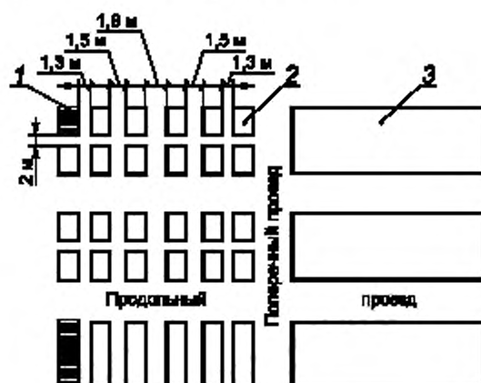
1 — пакет; 2 — штабель; 3 — группа штабелей
