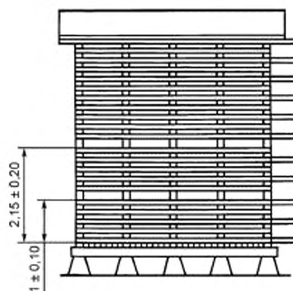
Рисунок А.9 — Горизонтальные каналы в рядовом штабеле
