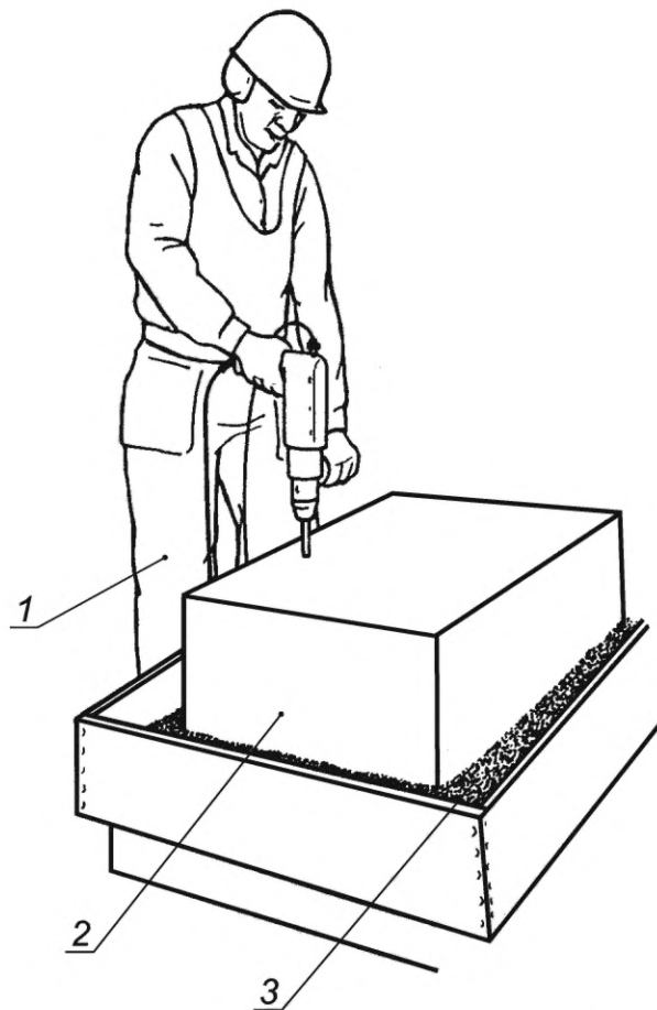
1 — оператор, стоящий на устройстве для измерения усилия, прилагаемого к инструменту; 2 — бетонный блок; 3 — упругий материал
