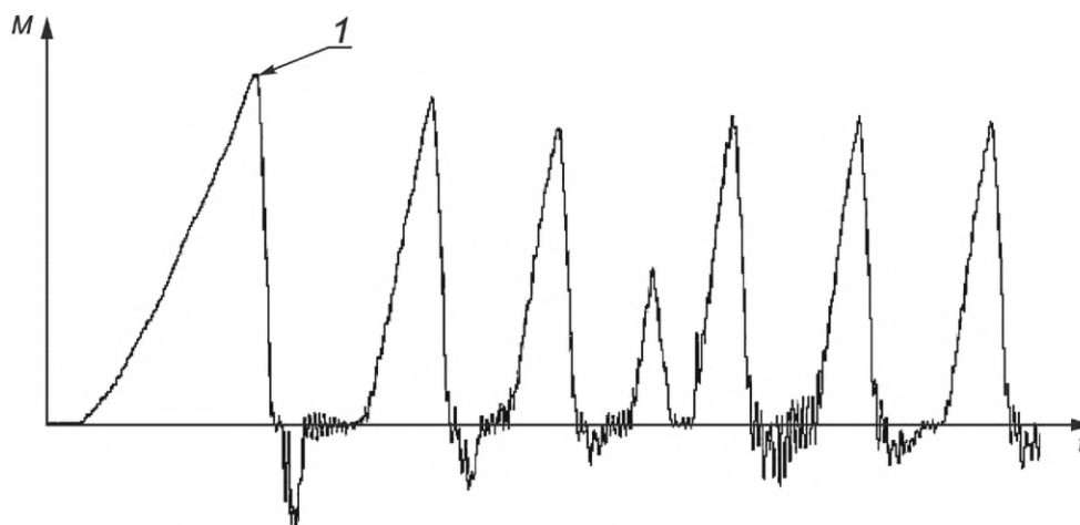
Рисунок 109 — Пример крутящего момента машины без стабильной области сигнала
