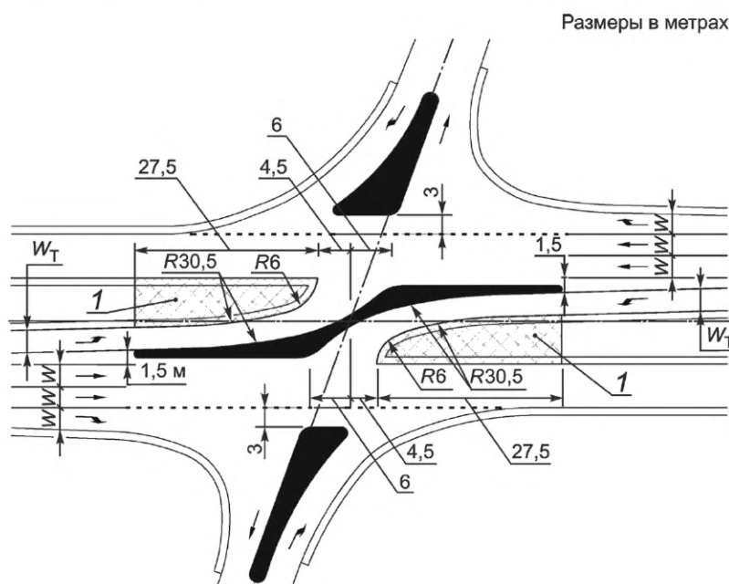
Рисунок 19 — Пересечение в одном уровне с отнесенными левыми поворотами с второстепенной дороги и левым поворотом с главной дороги без обеспечения прямого проезда по второстепенному направлению
