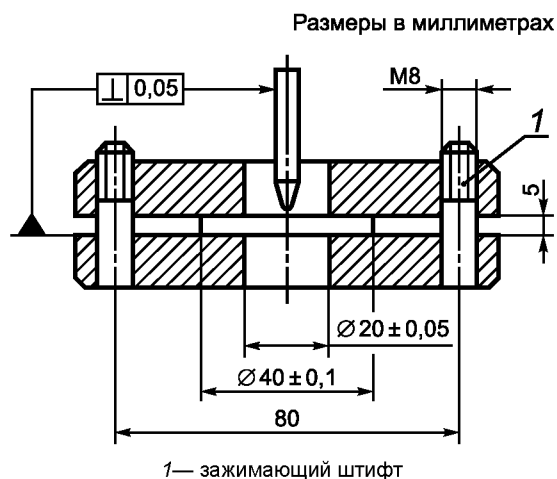
Рисунок 9— Удерживающее устройство
