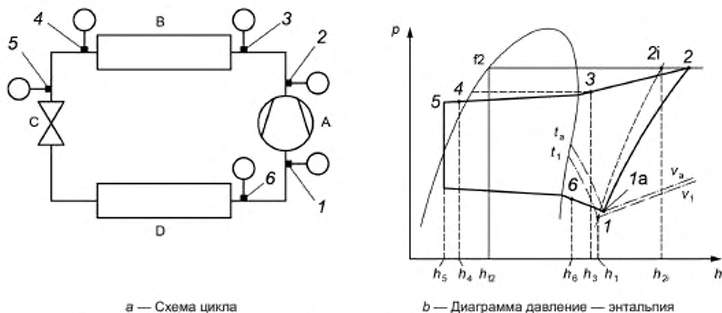
а — Схема цикла
