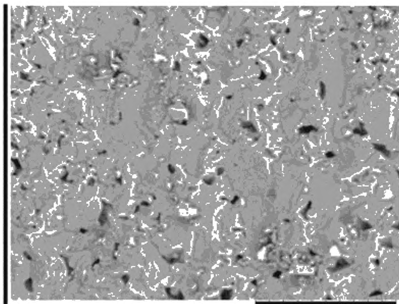
Рисунок А.1 — Микрофотография зеренной структуры керамики NKCNO-1. Маркер — 30 мкм
