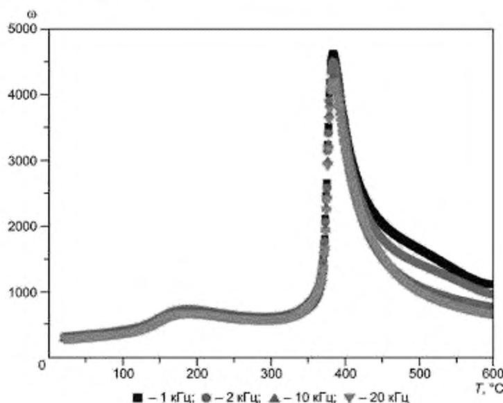
Рисунок А.2 — Зависимости \epsilon'/\epsilon_0(T) и \epsilon''/\epsilon_0(T) в частотном интервале f = (1 + 20) кГц
