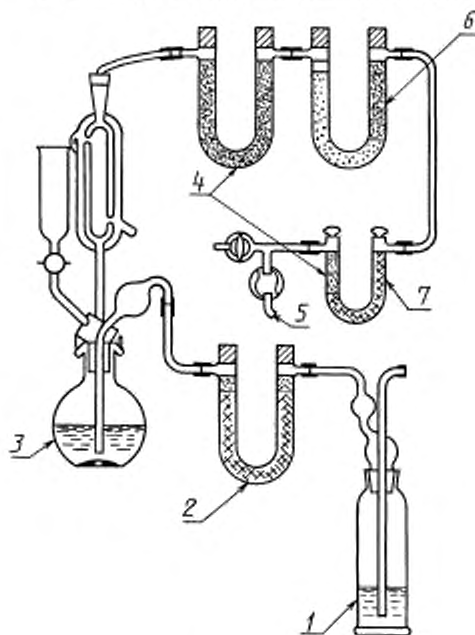
Установка для определения диоксида углерода
