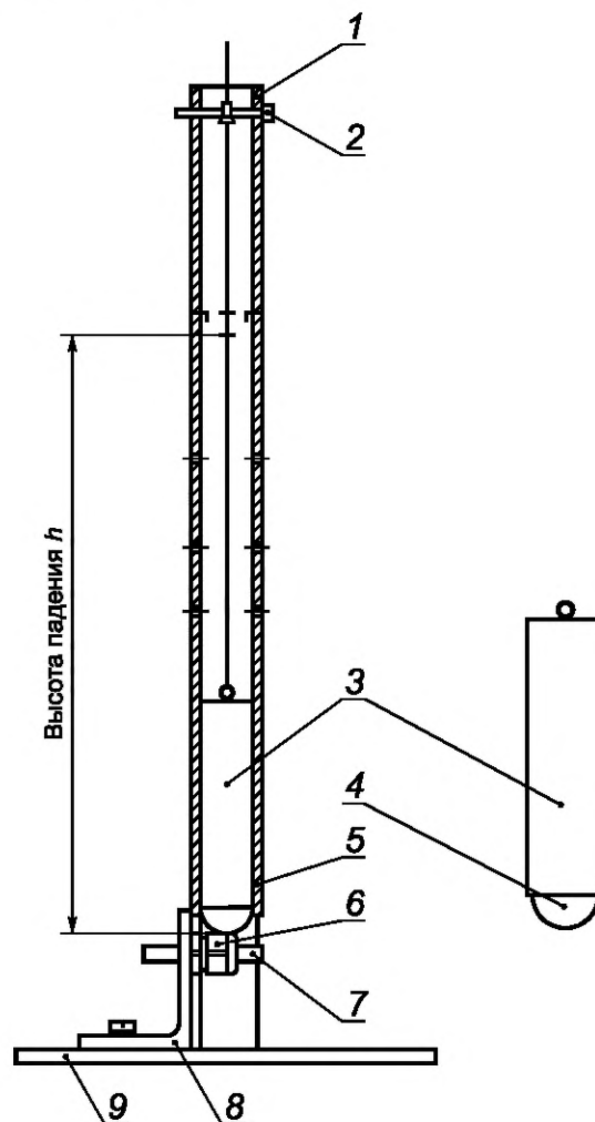
Рисунок А.3 — Пример испытательной установки на ударостойкость
