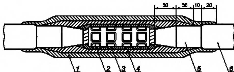
1 — самовулканизирующаяся полупроводящая лента; 2 — соединительная гильза; 3 — самовулканизирующаяся полупроводящая лента (для кабеля 6 кВ); 4 — самовулканизирующаяся изоляционная лента; 5 — изоляция жилы; 6 — экран по изоляции жилы
