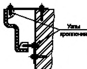
Рисунок 2 — Узел крепления СФБ изделия при вертикальной облицовке
