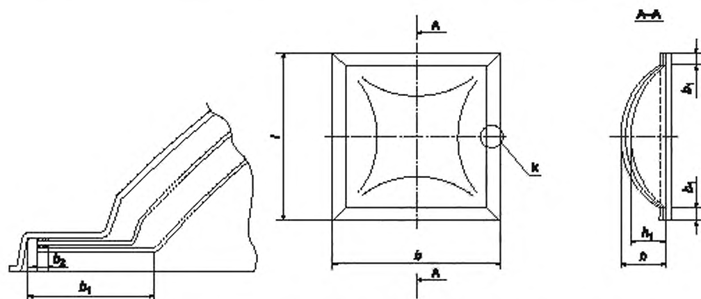
Рисунок А.2 — КПМ для установки с помощью винтовых прижимов (тип В)
