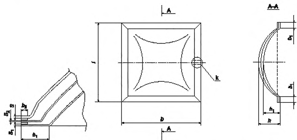
Рисунок А.3 — КРМ для установки с помощью рамы (тип Р)
