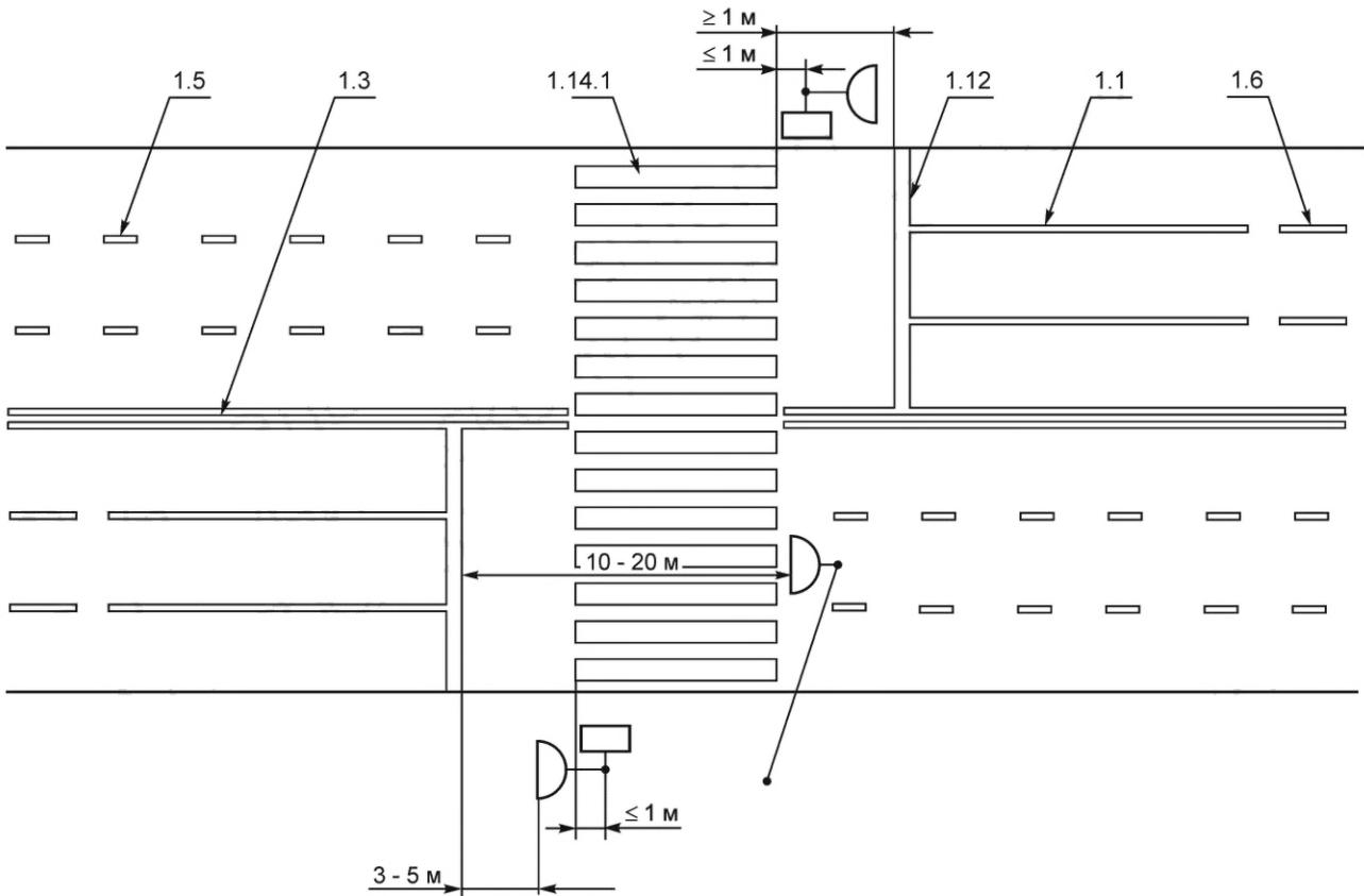
Рисунок В.20 — Пример размещения светофоров и нанесения разметки на регулируемом переходе
