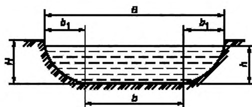
Рисунок 5 — Комбинированная форма поперечного сечения каналов проводящей сети
