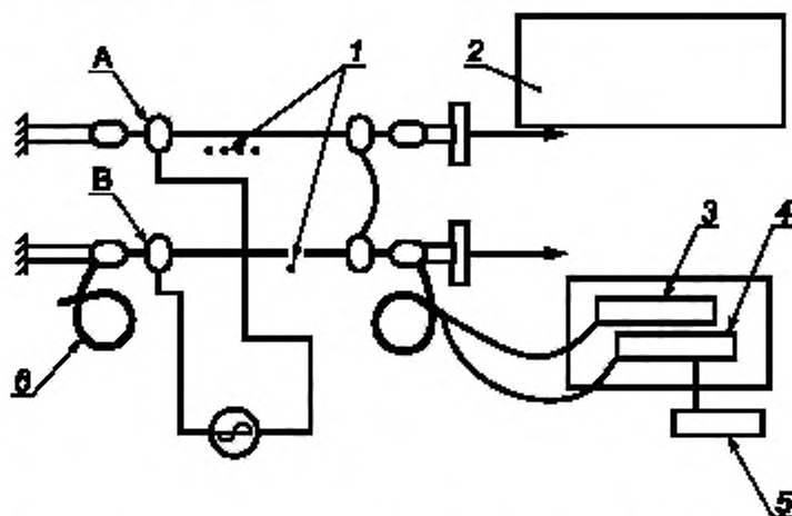
1 – датчики для измерения температуры: проволок, оптического модуля; 2 – устройство регистрации температуры; 3 – источник оптического излучения; 4 – измеритель оптической мощности; 5 – регистрирующее устройство. б – шлейф ОВ; А, В – испытуемые образцы
