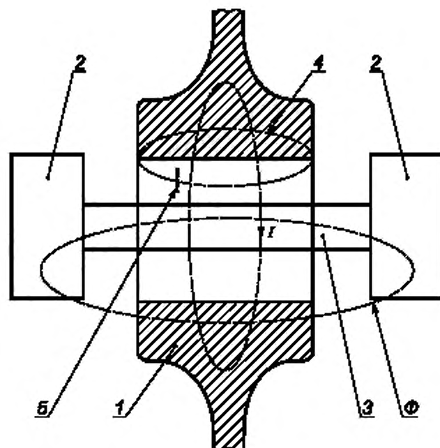
1 — цельнокатаное колесо; 2 — электромагнит; 3 — проводник; 4, \Phi — магнитные потоки, 5 — дефект; I — индуцированный ток
