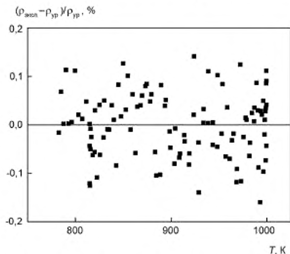
Рисунок 1 — Отклонение опытных данных настоящей работы о плотности жидкого сплава литий-свинец с содержанием 40,11 ат. % Pb от значений, рассчитанных по уравнению (1)
