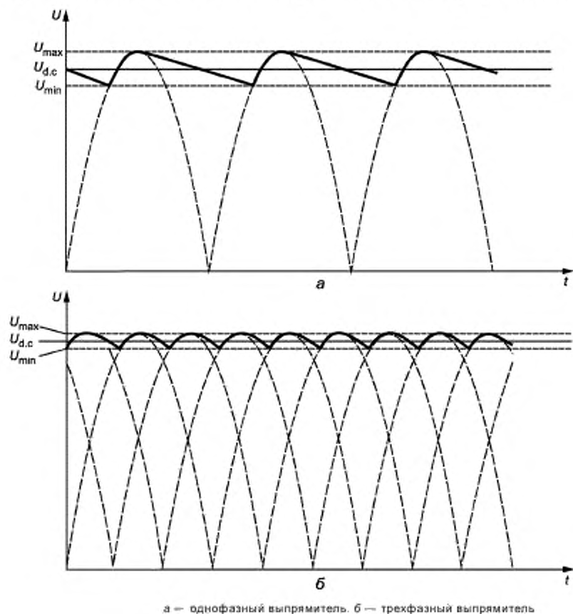
Рисунок 1 — Форма пульсаций напряжения
