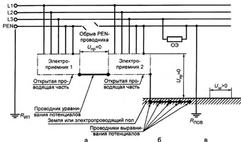
Рисунок В.2 — Сеть TN-C с оборванным PEN-проводником
