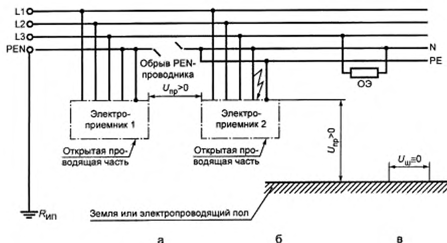
Рисунок В.7 — Сеть TN-C-S с обрывом PEN-проводника
