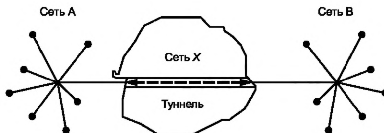
Рисунок 2 —Туннелирование
